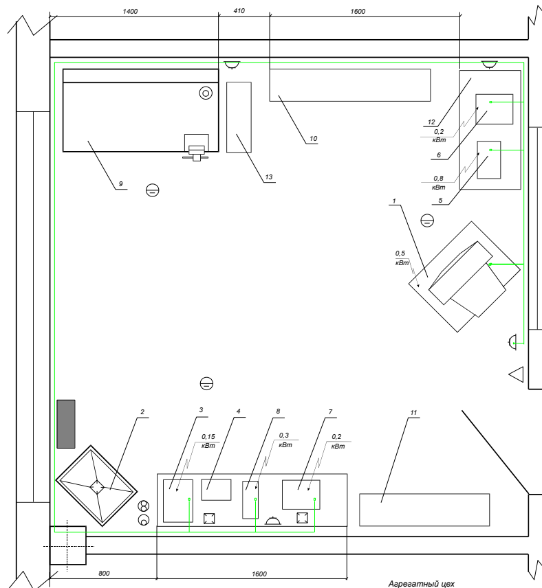
Рис. 1.1. Планировка Участка
