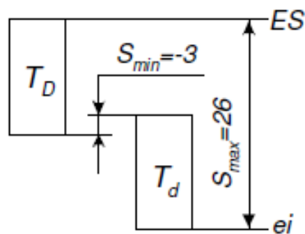
Рис. 2. Схема посадки.
