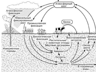
Рис. 1. – Схема круговорота азота в природе
