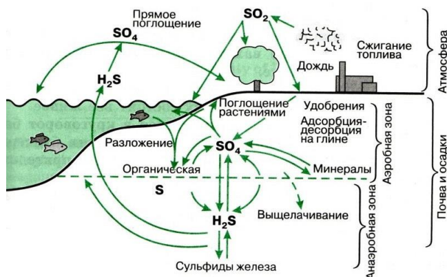
Рис. 3. – Схема круговорота серы в природе
