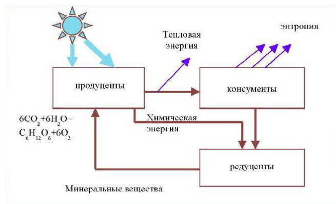
Рис. – Потоки вещества и энергии в экосистеме
