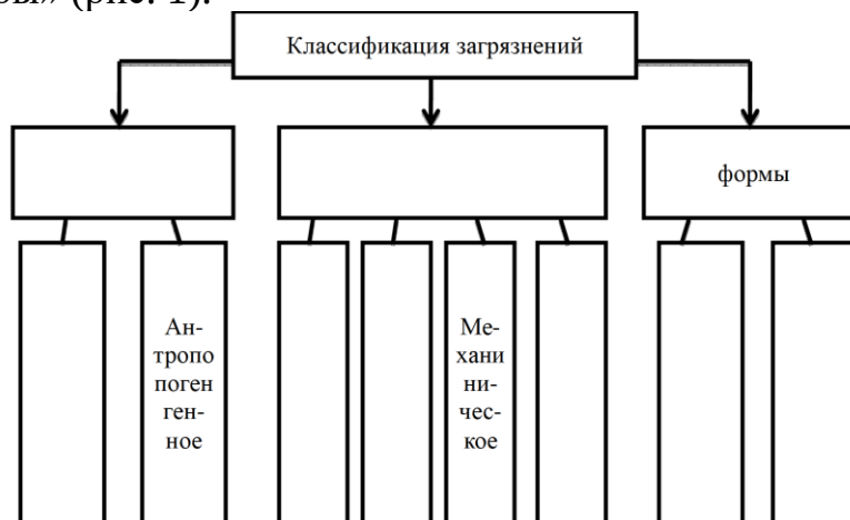
Рис 1. Классификация загрязнений биосферы.
