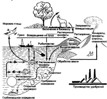
Рис. 2. – Схема круговорота фосфора в природе
